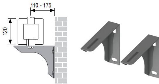
EWG25.001 - крепеж распределительного коллектора SMARTBOX 6.5
